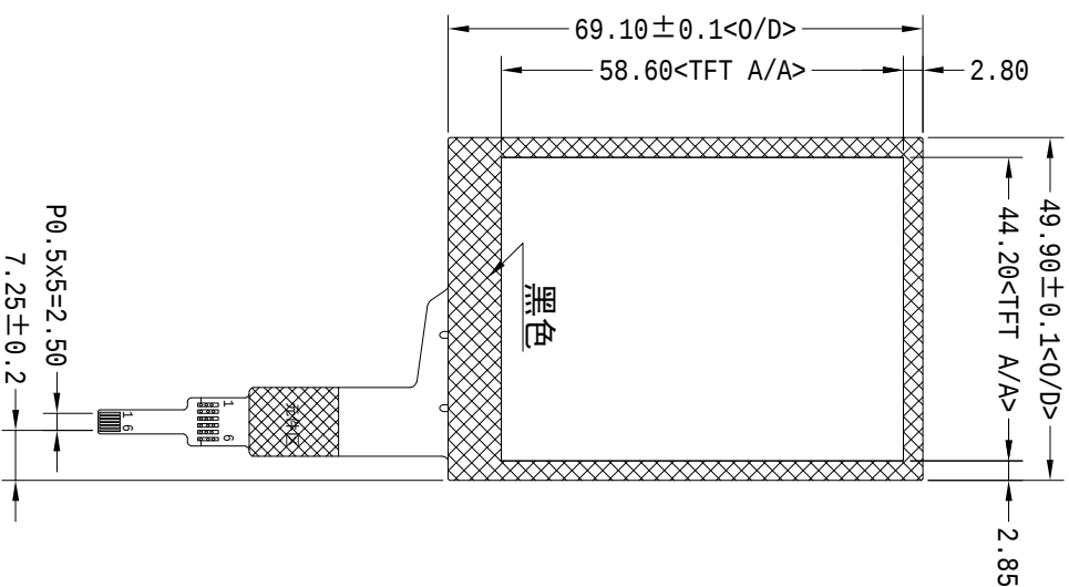
正视图 Front view
